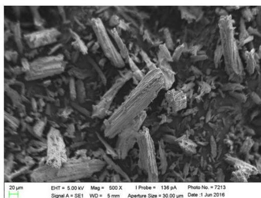
Figura 29 – Micrografias da fibra de sisal: in natura (a,c,e) e tratada (b,d,f)
