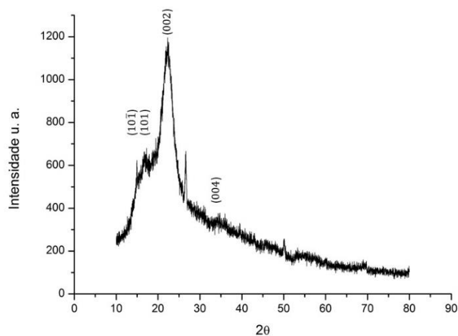
Figura 26 – DRX da fibra de sisal in natura
