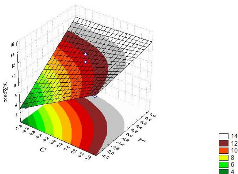
Figura 24 – Superfície de resposta para a concentração de xilose no pré-tratamento ácido da fibra de sisal
