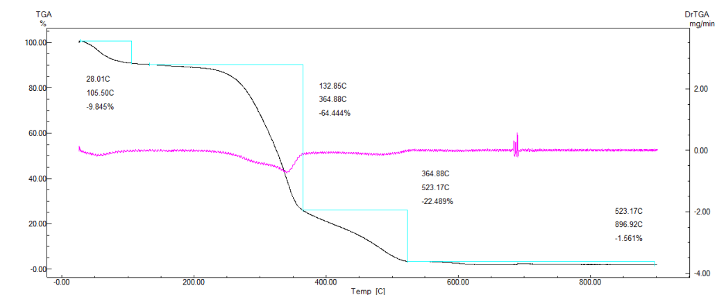
Figura 30 – Curva TG da fibra de sisal in natura em atmosfera de nitrogênio
