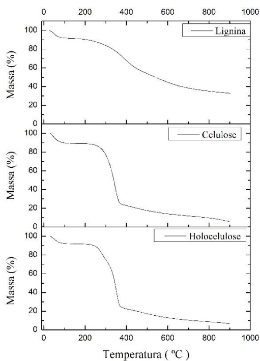
Figura 33 – Curvas TG dos constituintes da fibra de sisal em atmosfera de nitrogênio
