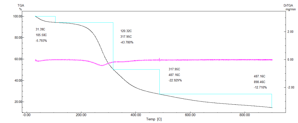
Figura 31 – Curva TG da fibra de sisal tratada em atmosfera de nitrogênio
