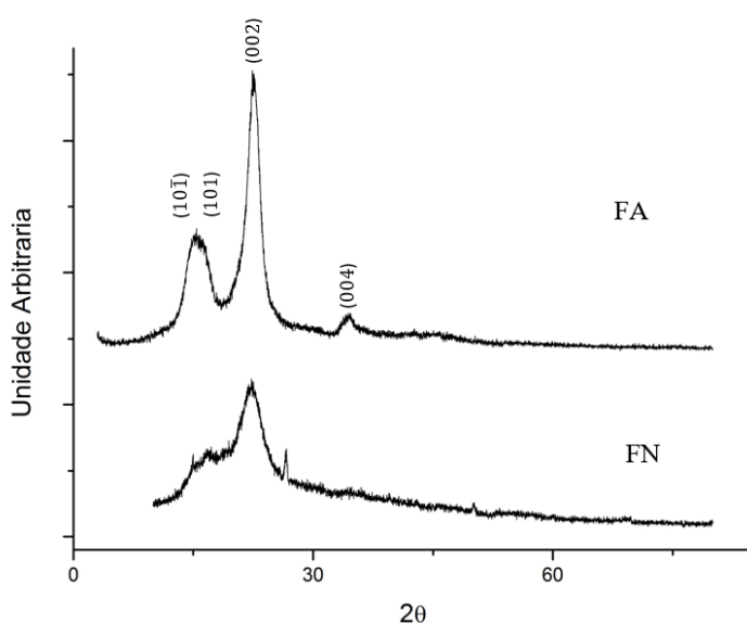
Figura 28 – Difratograma da fibra de sisal in natura (FN) e após o tratamento ácido (FA)
