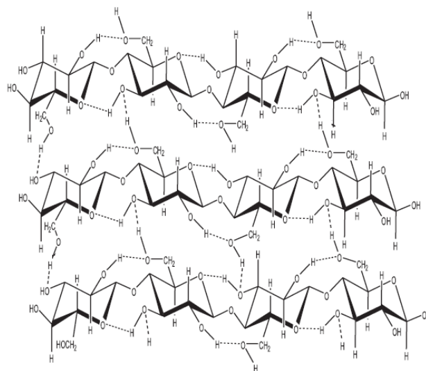
Figura 8 – Rede supramolecular da celulose
