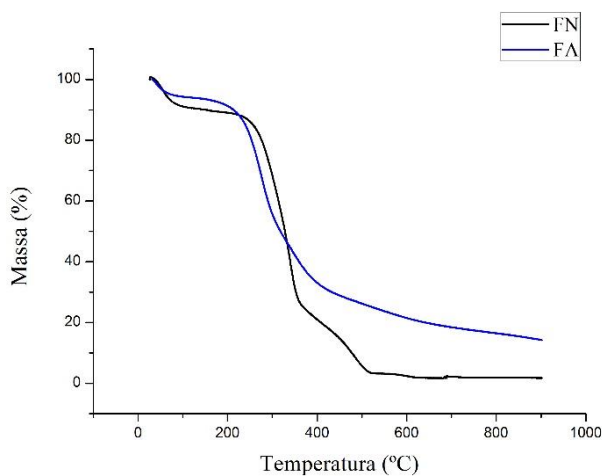
Figura 32 –Curvas TG da fibra de sisal in natura e tratada
