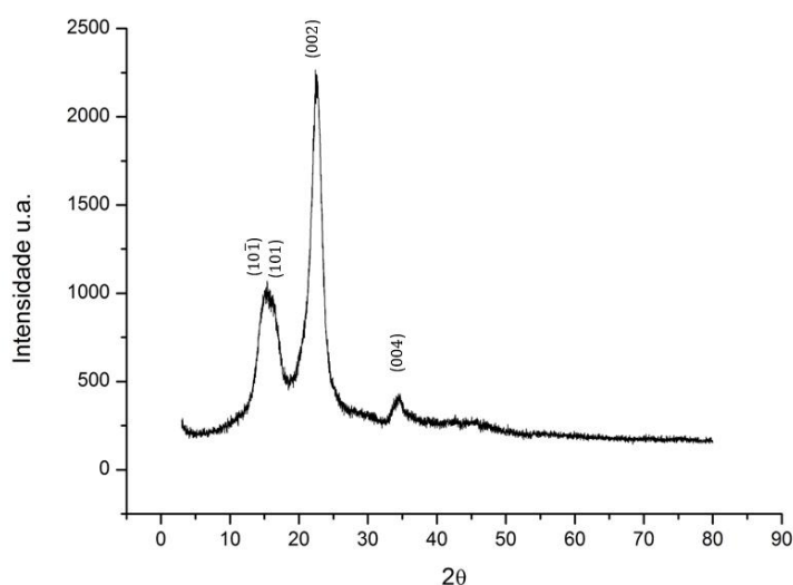
Figura 27 – DRX da fibra de sisal tratada
